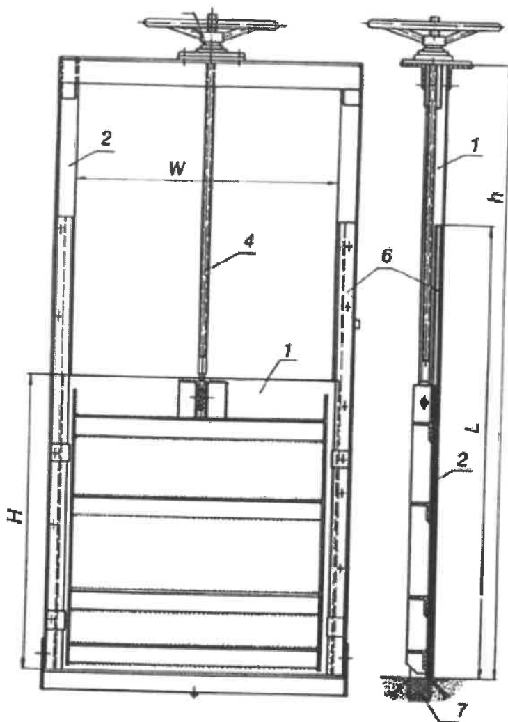
Slika 3: Zapornički mehanizam
